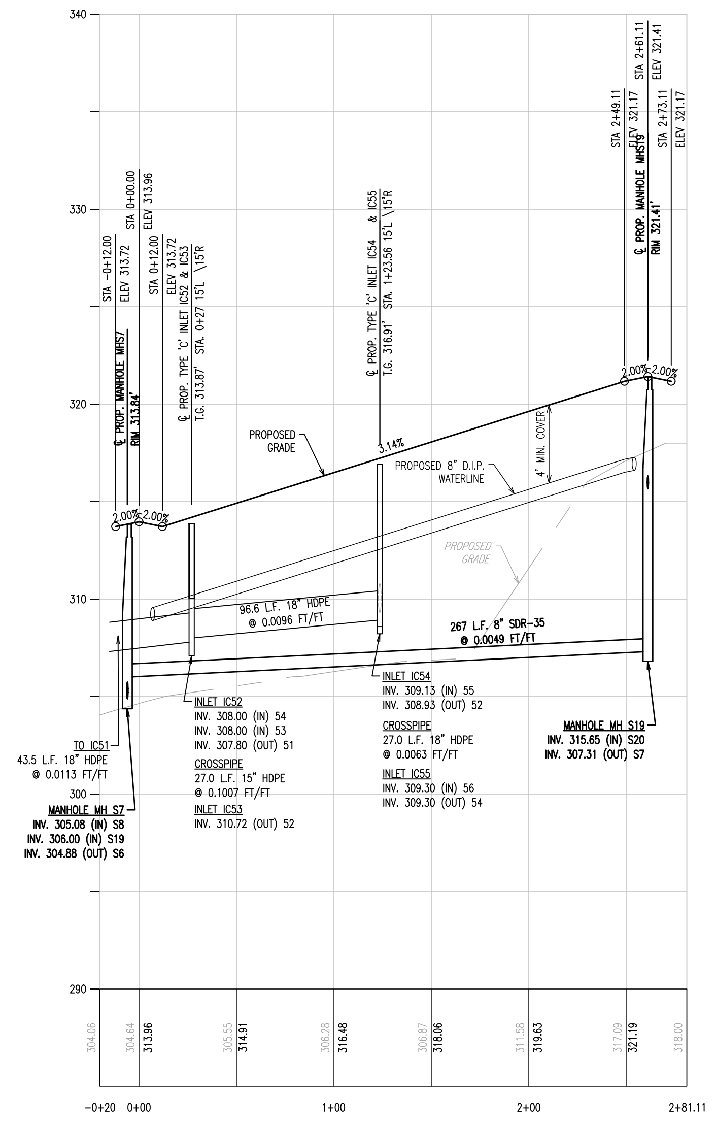
DRIVE 3 PROFILE STA -0+20 - 2+81.11 HORIZ SCALE: 1"=50' VERT SCALE: 1"=5'
