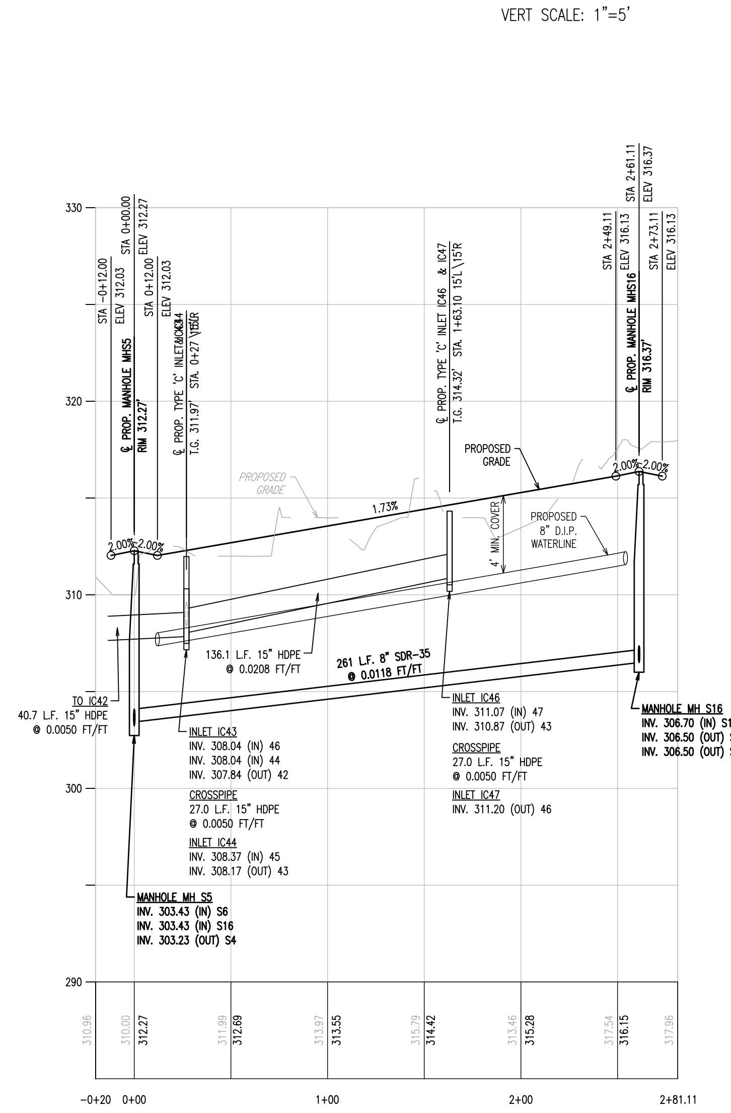
DRIVE 2 PROFILE STA -0+20 - 2+81.11 HORIZ SCALE: 1"=50' VERT SCALE: 1"=5'
