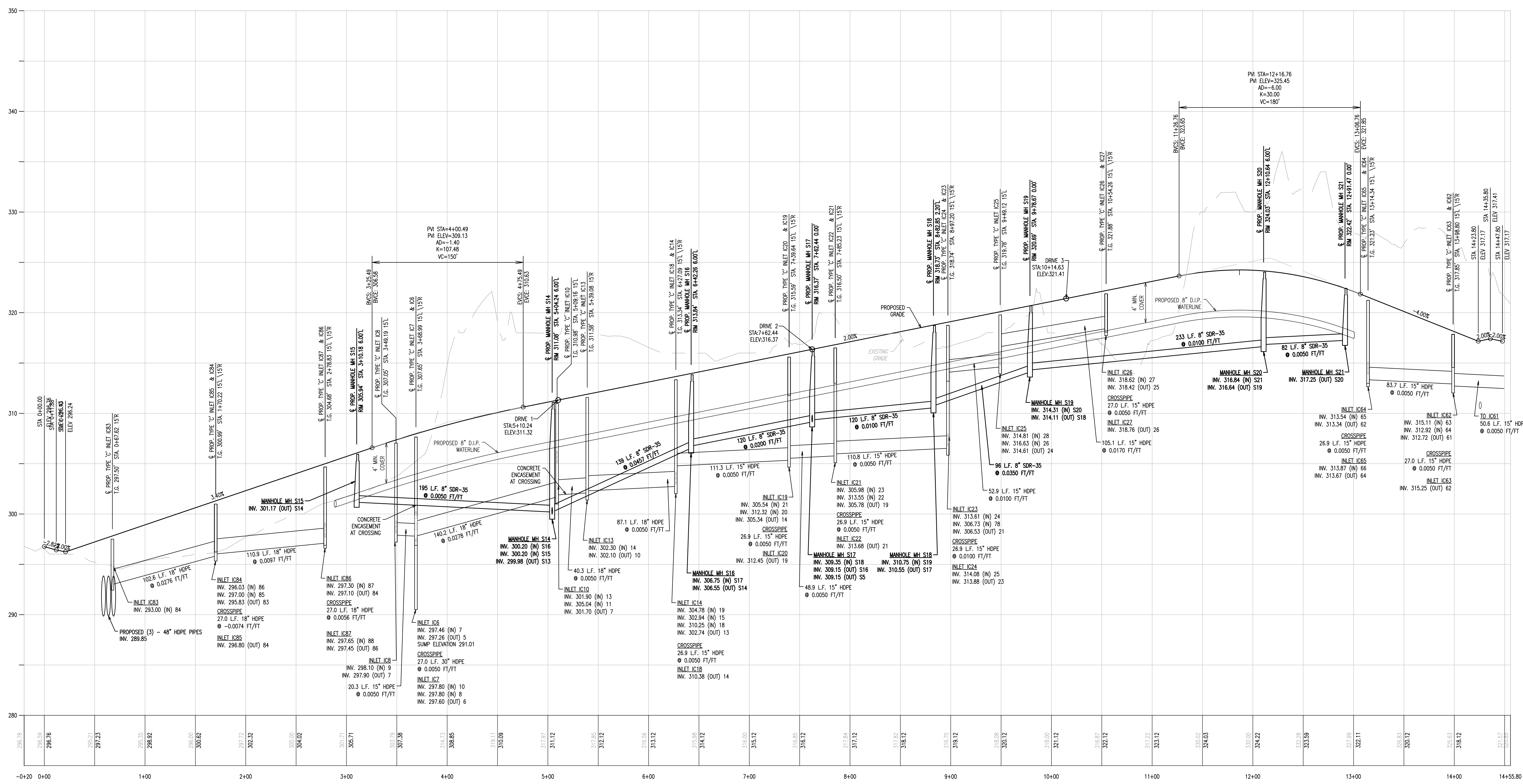
INTERNAL DRIVE B PROFILE STA -0+20 - 14+55.80 HORIZ SCALE: 1"=50' VERT SCALE: 1"=5'
