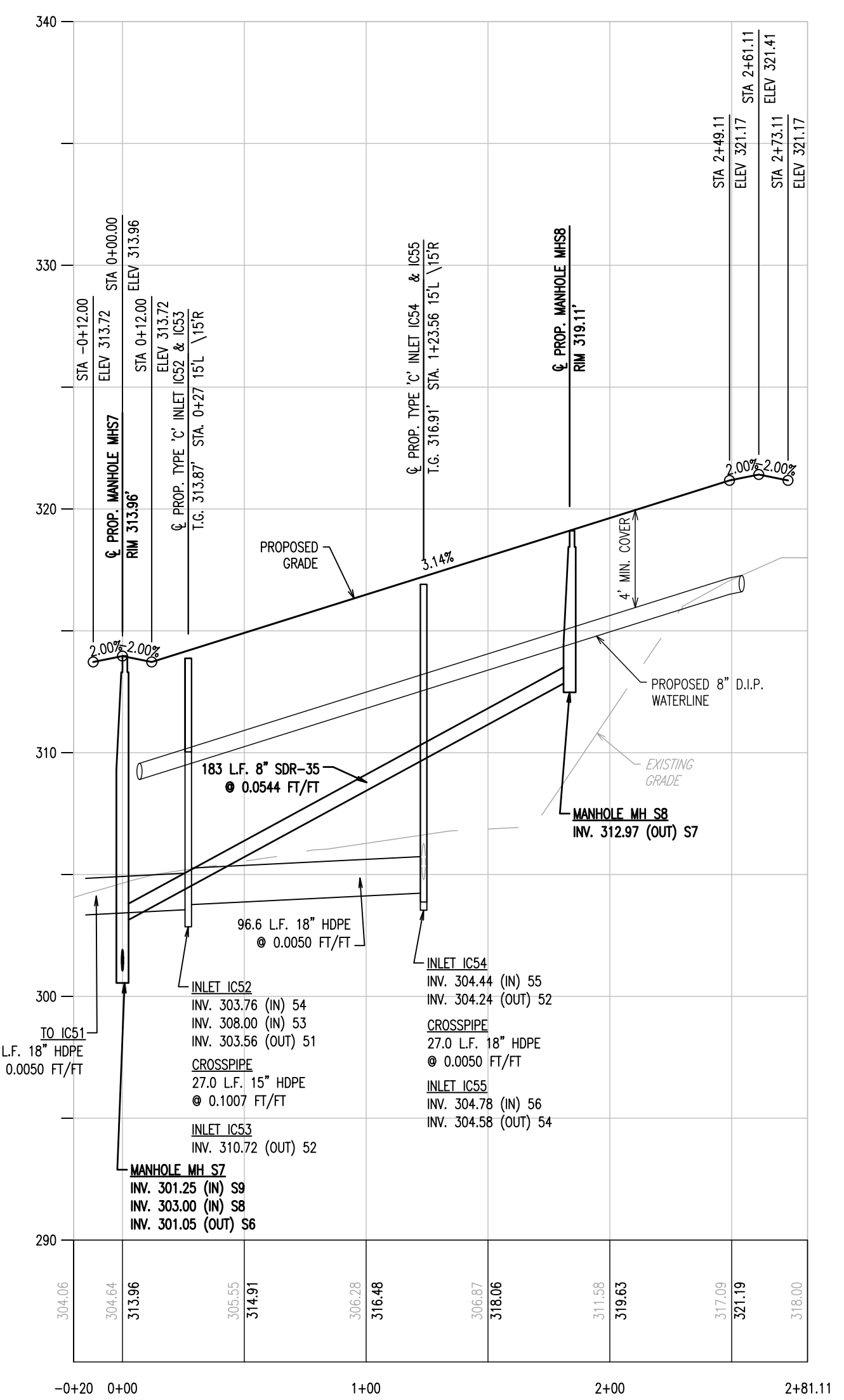
DRIVE 3 PROFILE STA -0+20 - 2+81.11 HORIZ SCALE: 1"=50' VERT SCALE: 1"=5'
