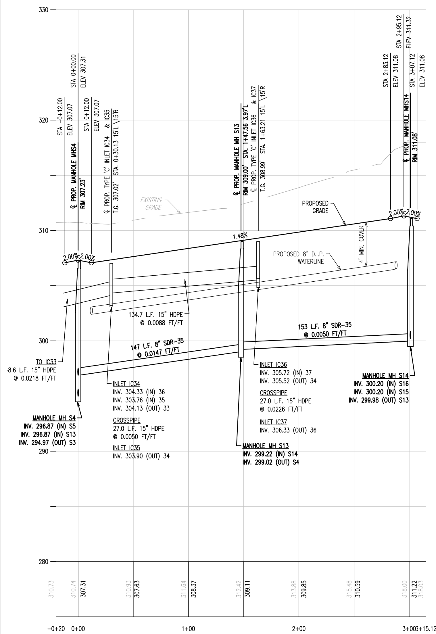
DRIVE 1 PROFILE STA -0+20 - 3+15.12 HORIZ SCALE: 1"=50' VERT SCALE: 1"=5'
