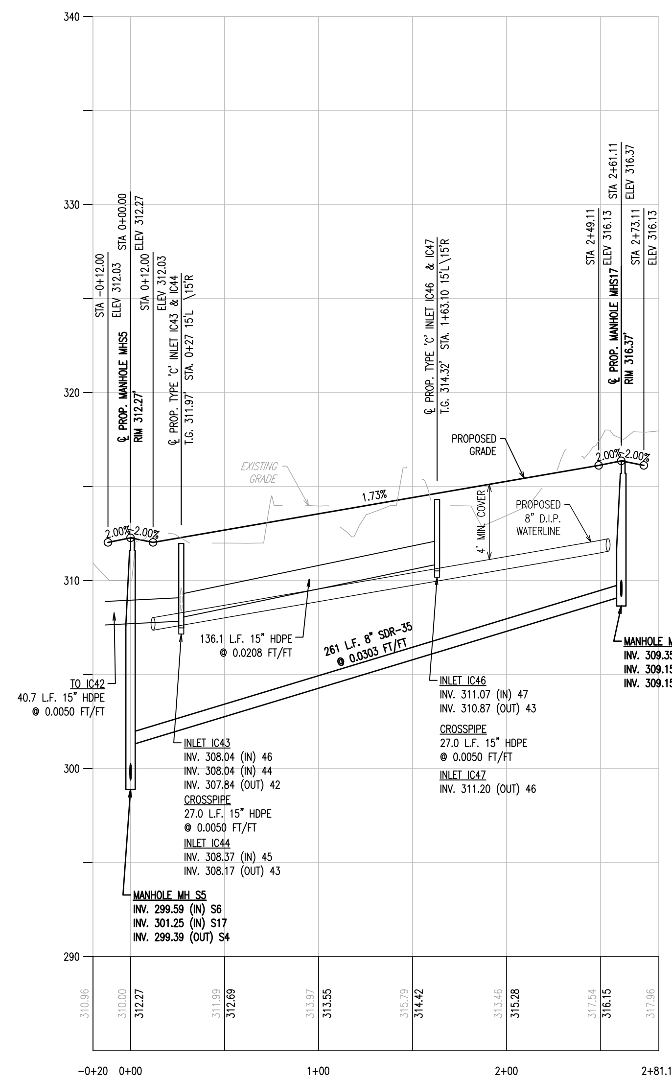
DRIVE 2 PROFILE STA -0+20 - 2+81.11 HORIZ SCALE: 1"=50' VERT SCALE: 1"=5'
